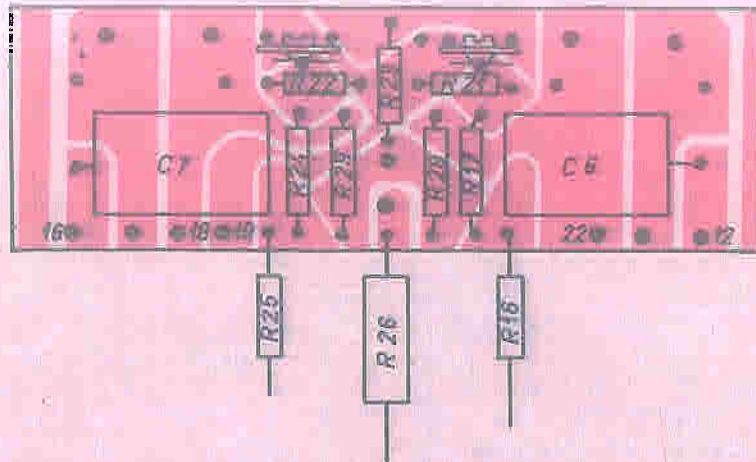
obr. 17. Deska předpětí pro koncový stupeň (pohled ze strany součástek)
